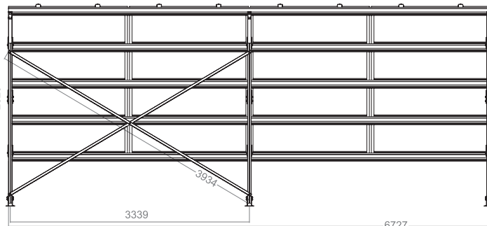
Back view of a triangle in 4 Landscape layout Izgled zadnjeg dela fotonaponskih panela
