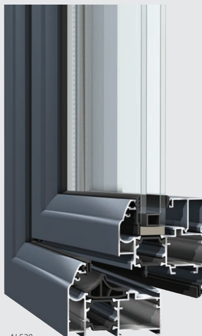
AL520 CE (Eurožleb)
