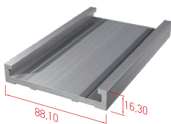
Base guide Sina nosača
