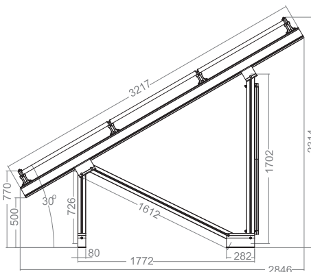
Side view of a triangle in 3 Landscape layout Bočni izgled fotonaponskih panela
