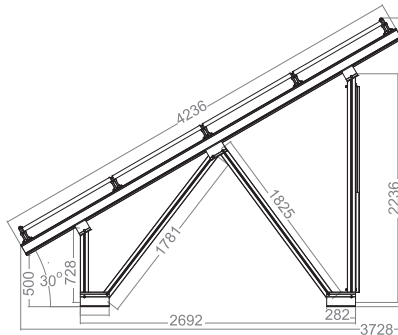
Side view of a triangle in 4 Landscape layout Bočni izgled fotonaponskih panela
