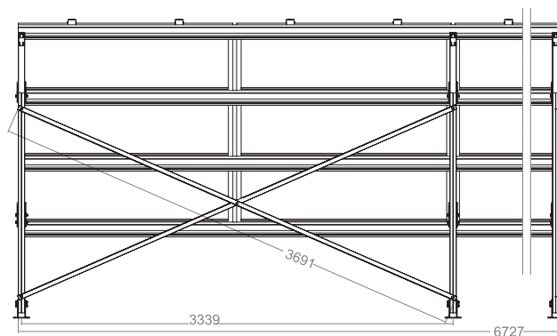
Back view of a triangle in 3 Landscape layout Izgled zadnjeg dela fotonaponskih panela
