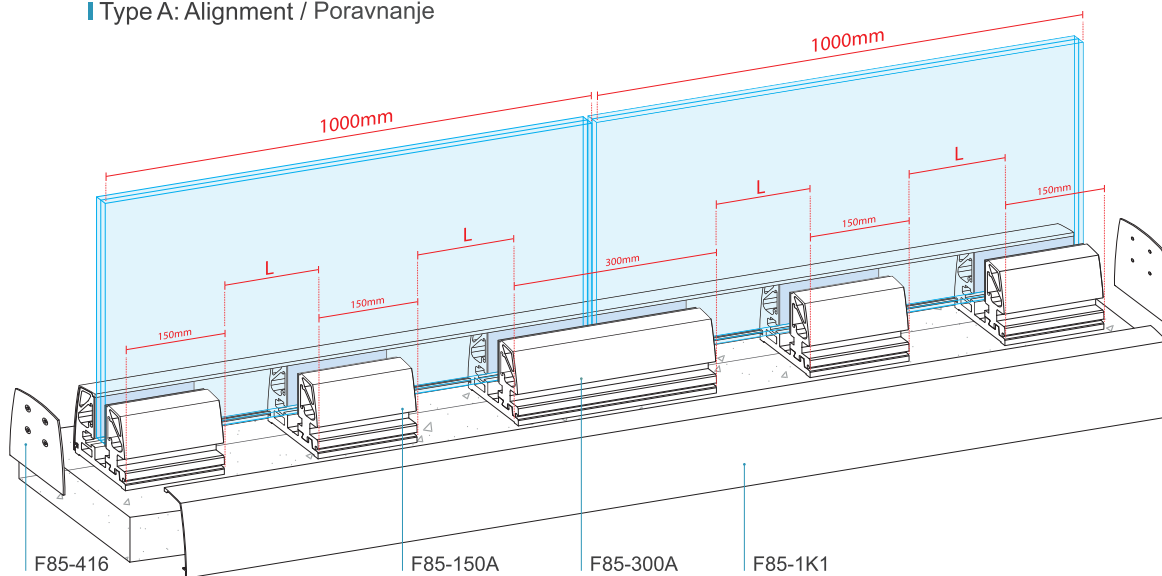
Type A: Alignment / Poravnanje
