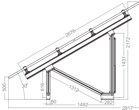
Side view of a triangle in 2 Portrait layout Bočni izgled fotonaponskih panela
