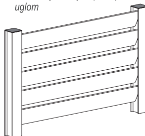
3 Internal curved rabote in angle Unutrašnji zaobljeni profil pod uglom
